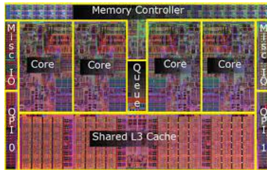
Fig. 1.1 Nehalem
